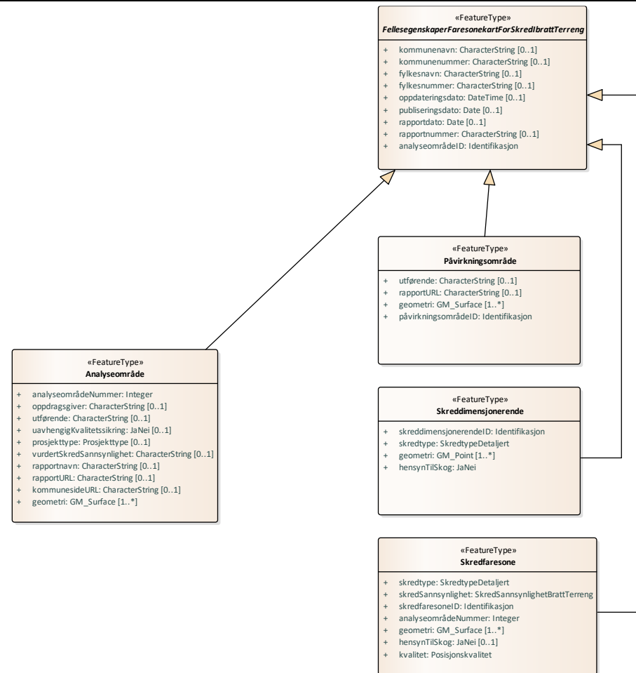
Figur 3: Realisering av objekttyper FaresonekartForSkredIbrattTerreng
