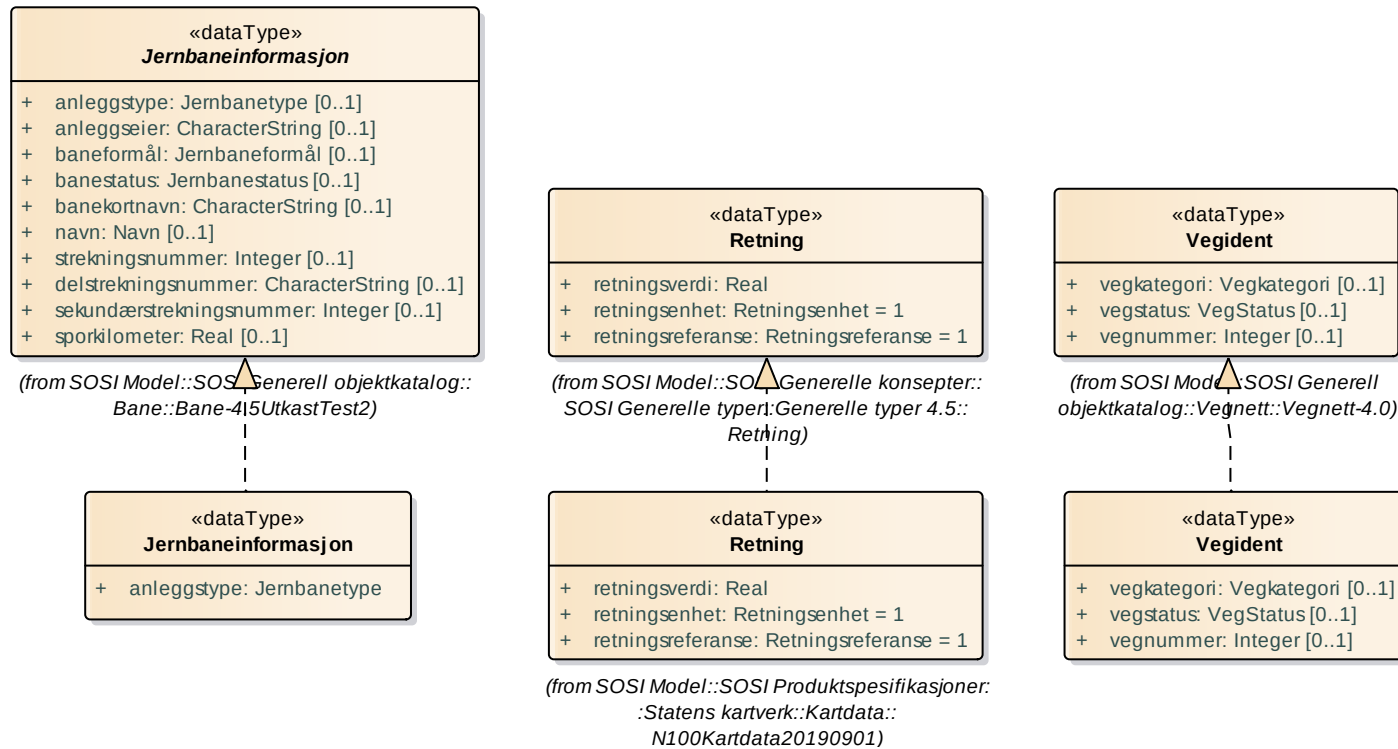
Figur 41 Realisering av datatyper fra generell objektkatalog
