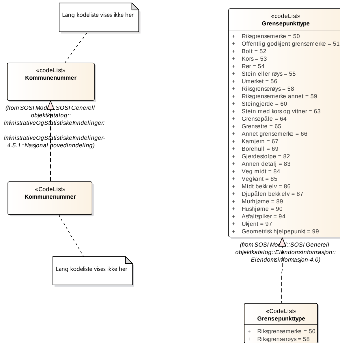
Figur 7 Realisering av kodelister fra generell objekt katalog
