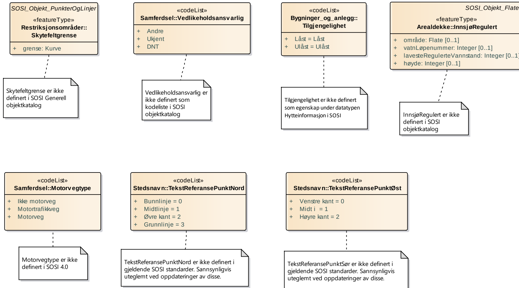
Figur 53 Utvidelser i forhold til SOSI del 1 og 2
