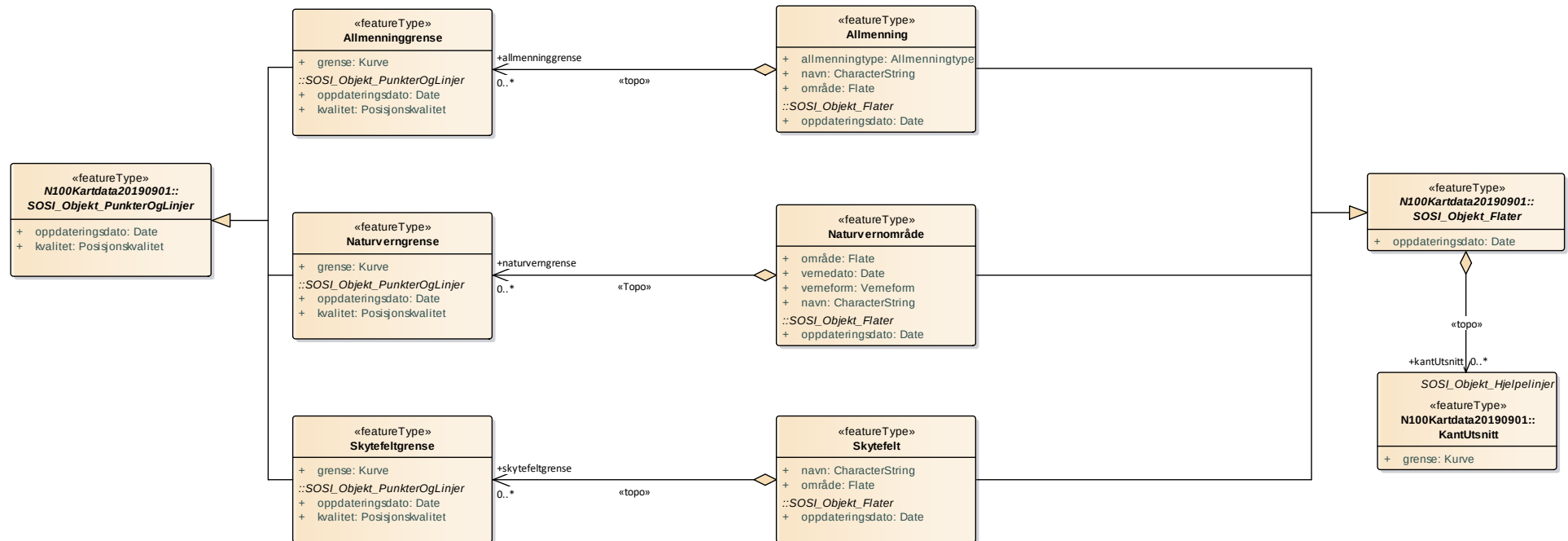
Figur 37 Restriksjonsområder
