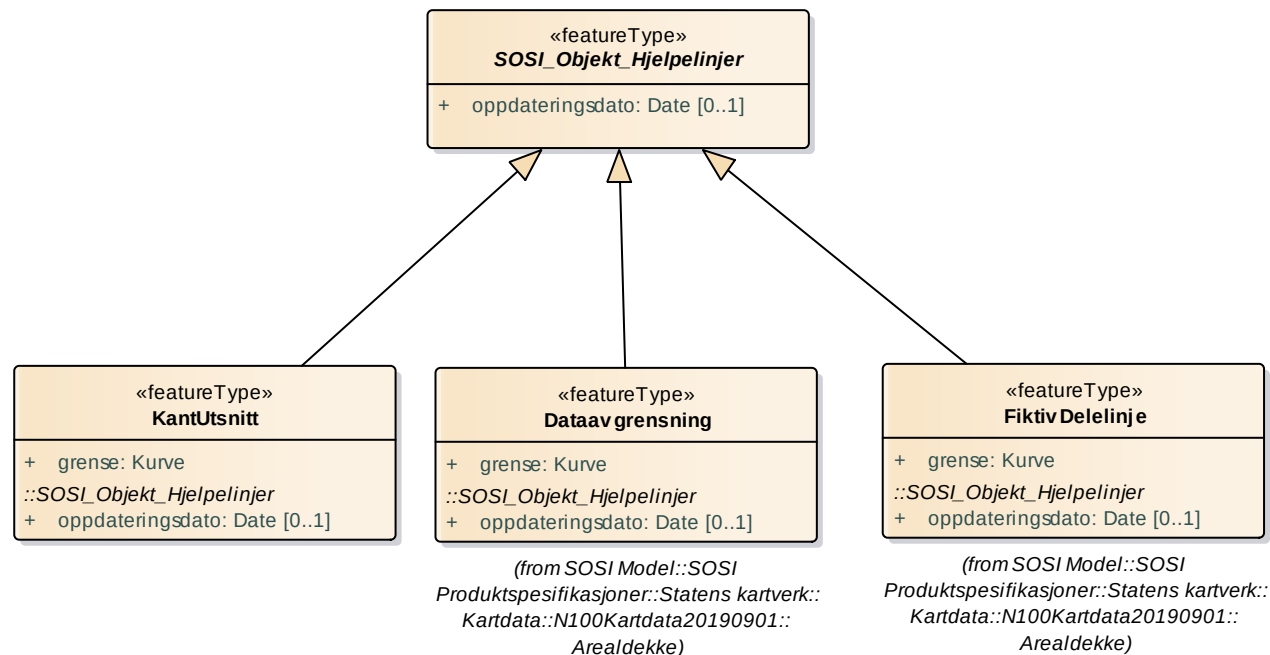
Figur 1 Hjelpelinjer
