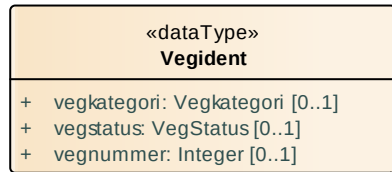
Figur 44 Datatyper
