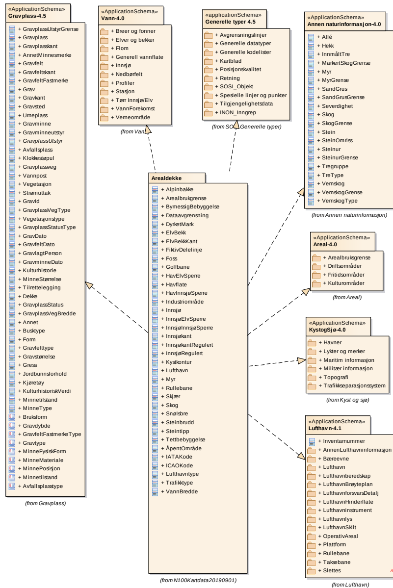
Figur 10 Pakkeavhengighet
