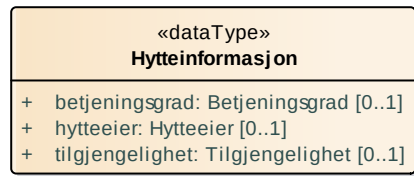
Figur 27 Datatyper
