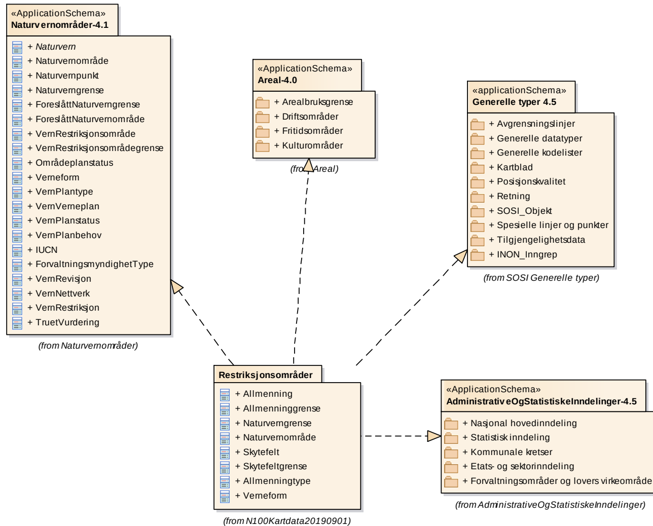
Figur 34 Pakkeavhengighet
