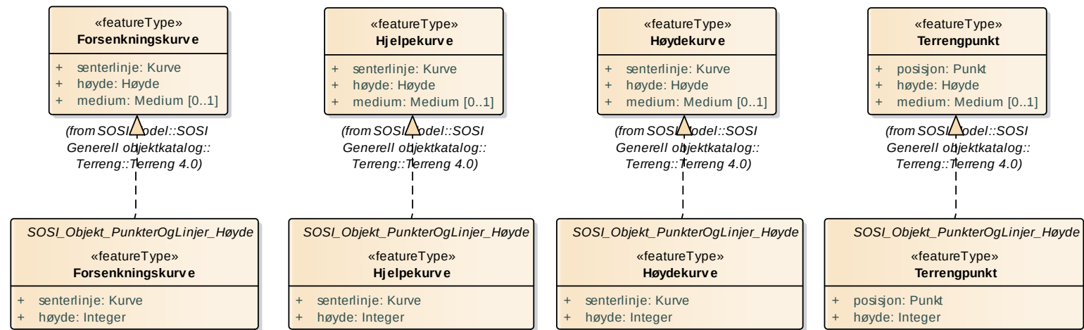
Figur 30 Realisering av featuretyper fra generell objektkatalog
