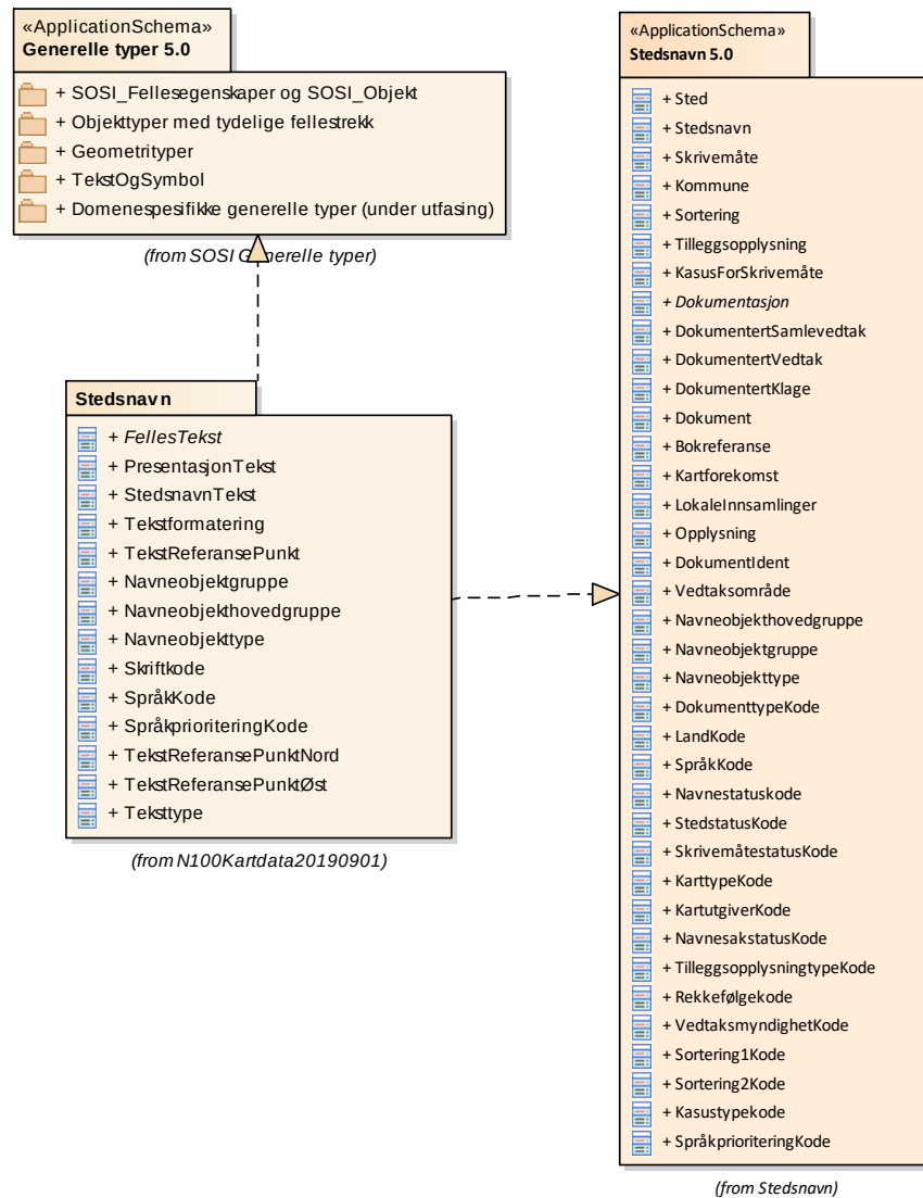
Figur 46 Pakkeavhengighet
