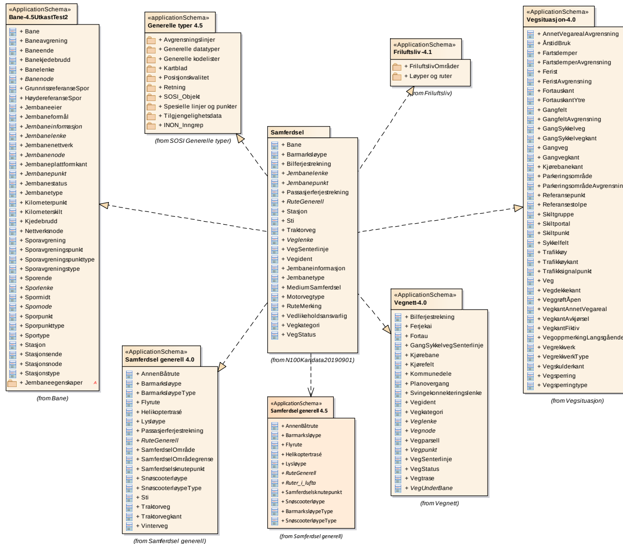
Figur 39 Pakkeavhengighet
