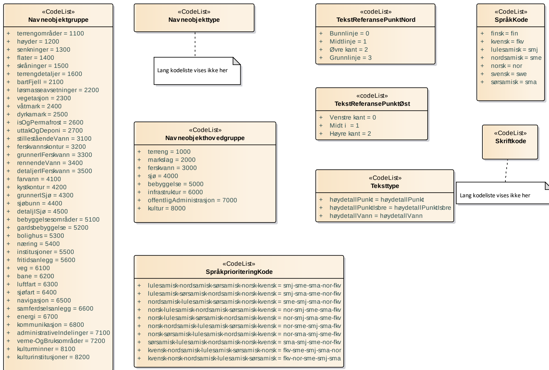
Figur 51 Kodelister
