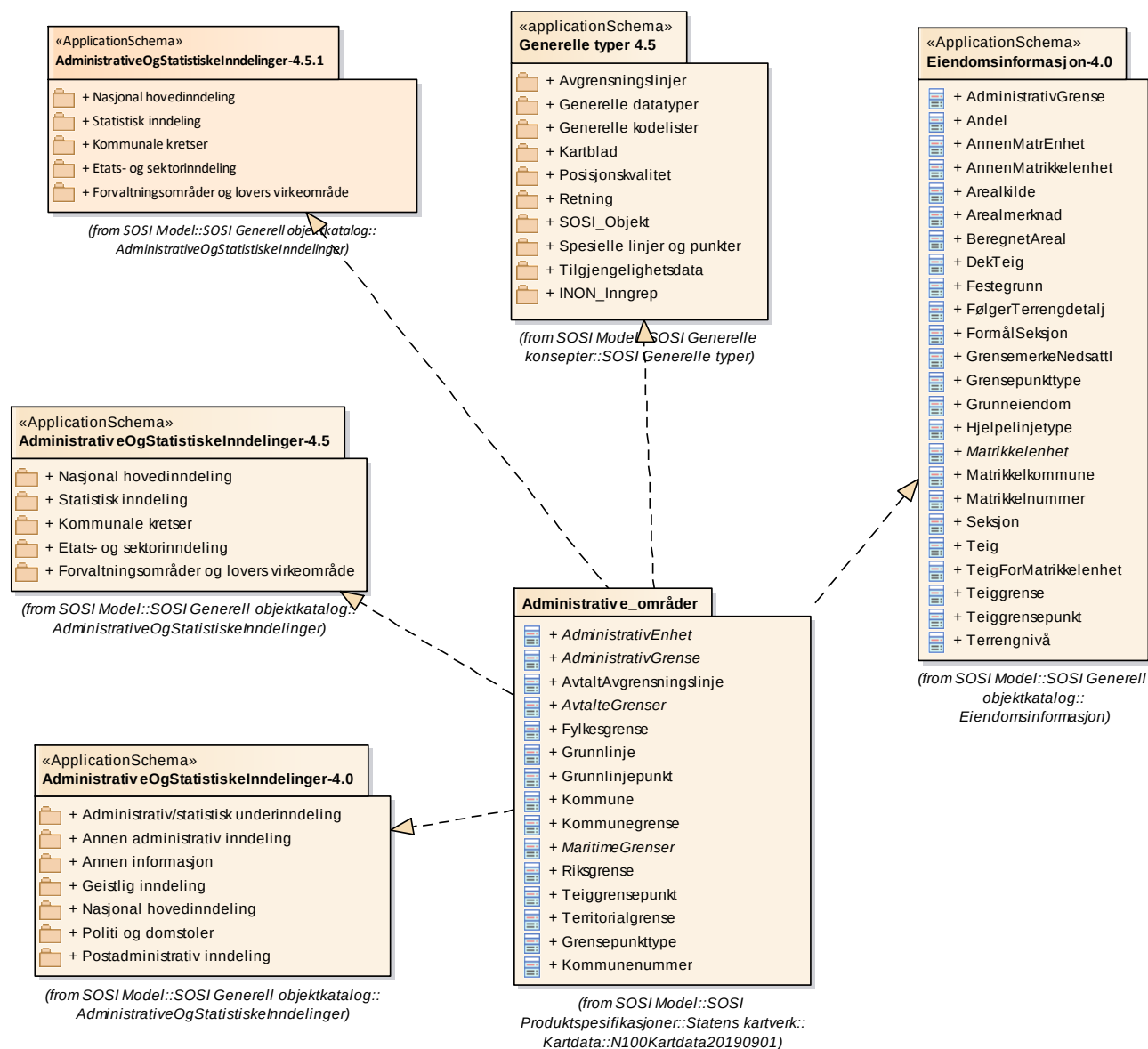
Figur 5 Pakkeavhengighet
