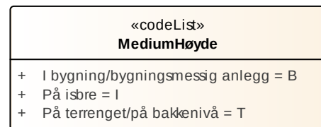
Figur 33 Kodelister
