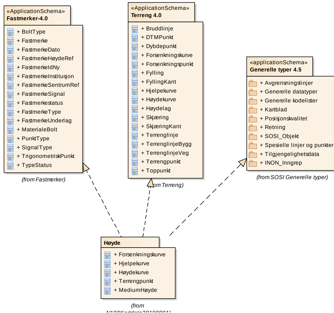
Figur 29 Pakkeavhengighet
