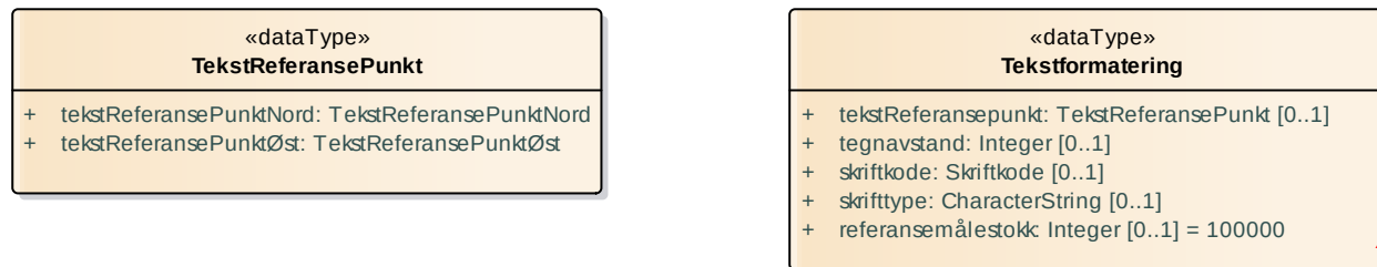
Figur 50 Datatyper
